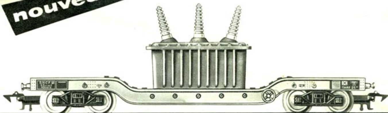
SURBAISSÉ Référence 658C
